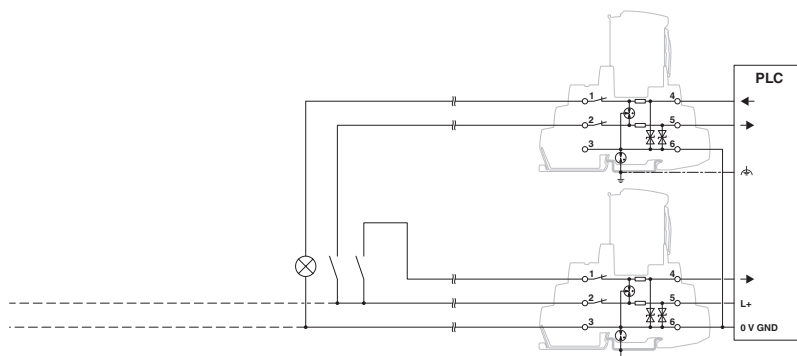
Applikasjonstegning
