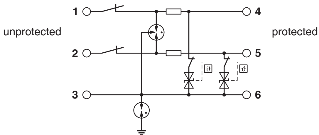
Koblingsskjema
