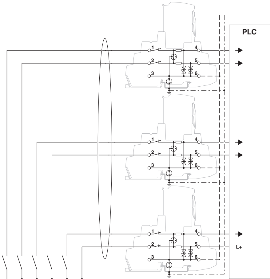
Applikasjonstegning
